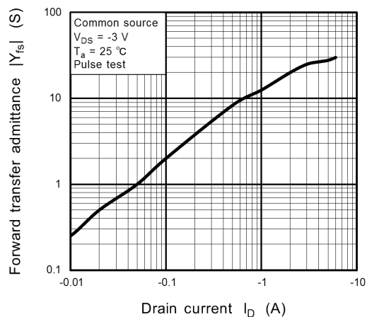
Fig. 7.7 |Y_{fs}| - I_D
