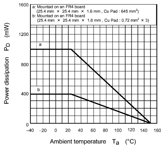
Fig. 7.13 P_D - T_a
