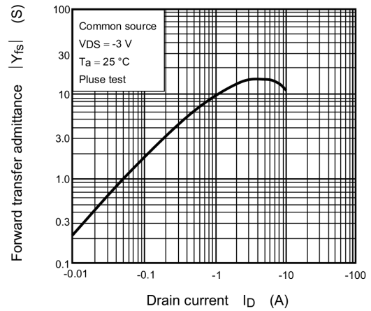
Fig. 7.8 |Y_{fs}| - I_D
