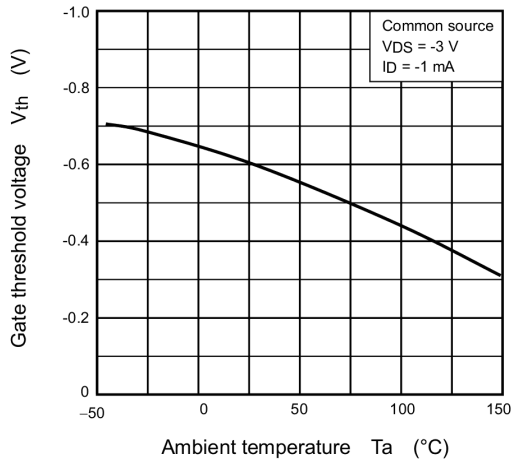
Fig. 7.7 V_{th} - T_a
