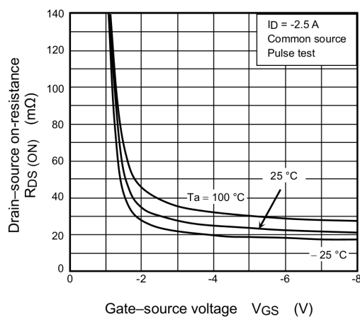
Fig. 7.4 R_{DS(ON)} - V_{GS}
