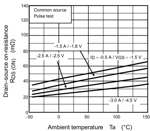
Fig. 7.6 R_{DS(ON)} - T_a
