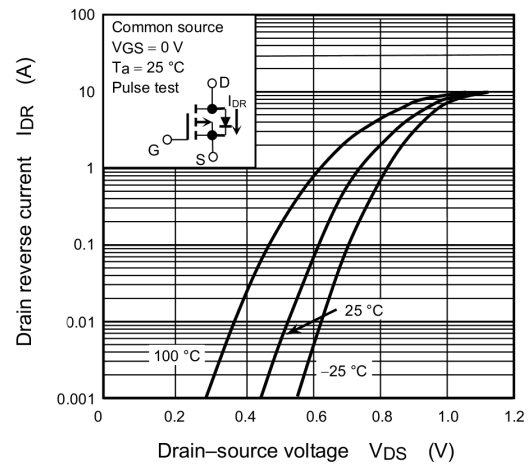
Fig. 7.12 I_{DR} - V_{DS}
