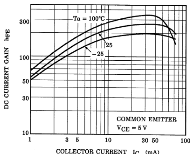
Fig. 10.16 RN1404 h_{FE}-I_C
