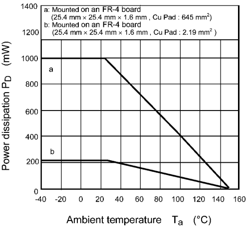
Fig. 7.14 P_D - T_a
