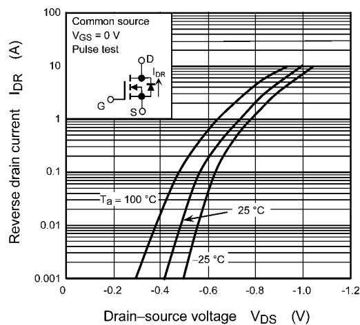
Fig. 7.9 I_{DR} - V_{DS}
