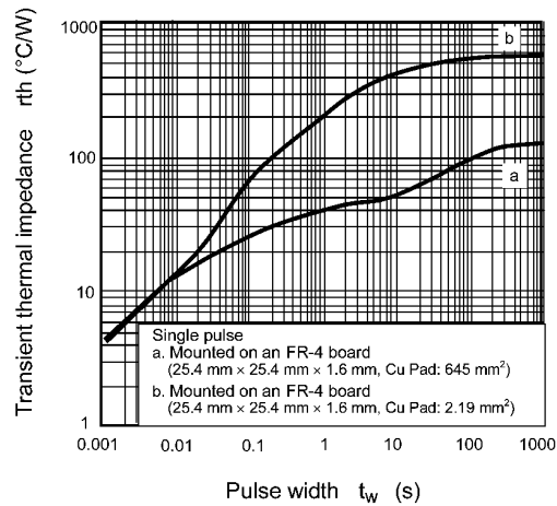
Fig. 7.13 r_{th} - t_w
