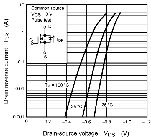
Fig. 7.8 I_{DR} - V_{DS}
