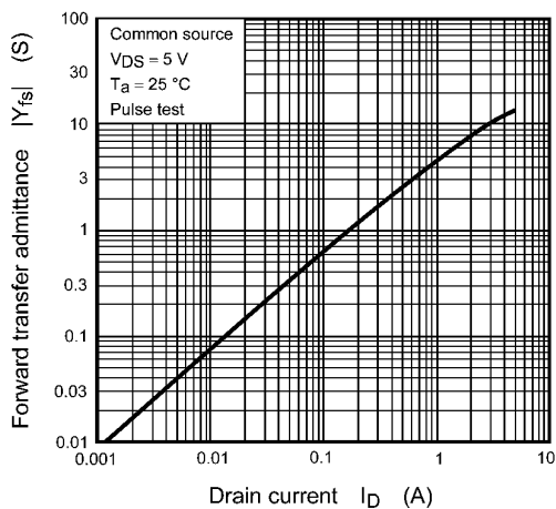
Fig. 7.7 |Y_{fs}| - I_D
