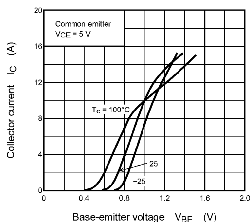
Fig. 8.4 I_C - V_{BE}
