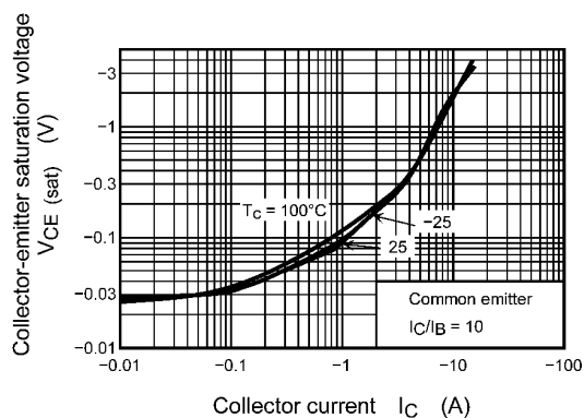
Fig. 8.1 I_C - V_{CE}
