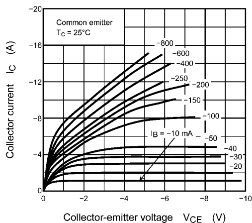
Fig. 8.1 I_C - V_{CE}
