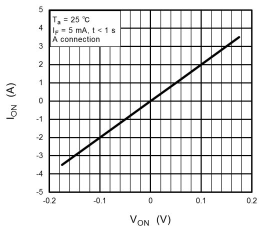
Fig. 13.1.4 I_{ON} - V_{ON}
