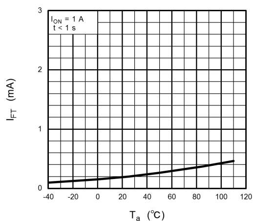
Fig. 13.1.6 I_{FT} - T_a
