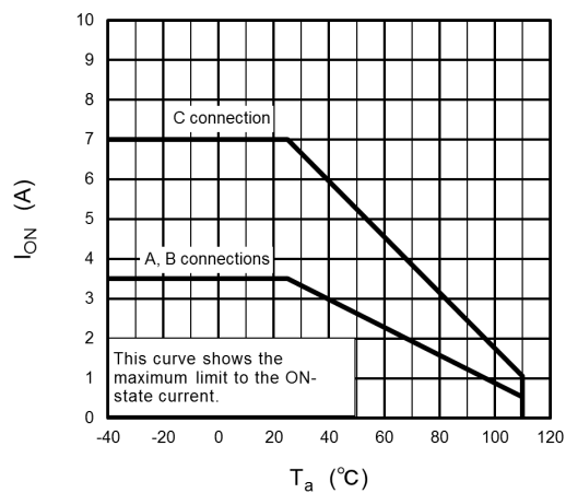
Fig. 13.1.2 I_{ON} - T_a
