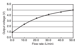
D6F-10A5-000
