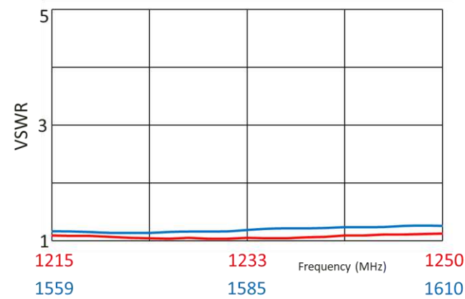
VSWR
