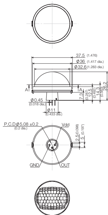
SECTION A-A
