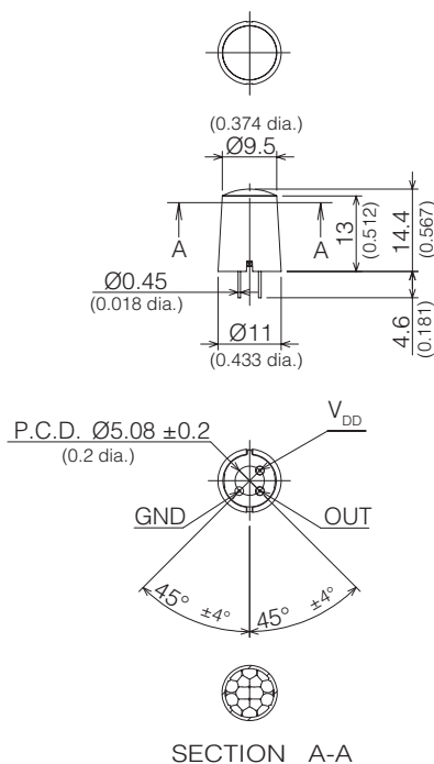
SECTION A-A
