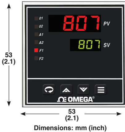
Bezel Dimensions
