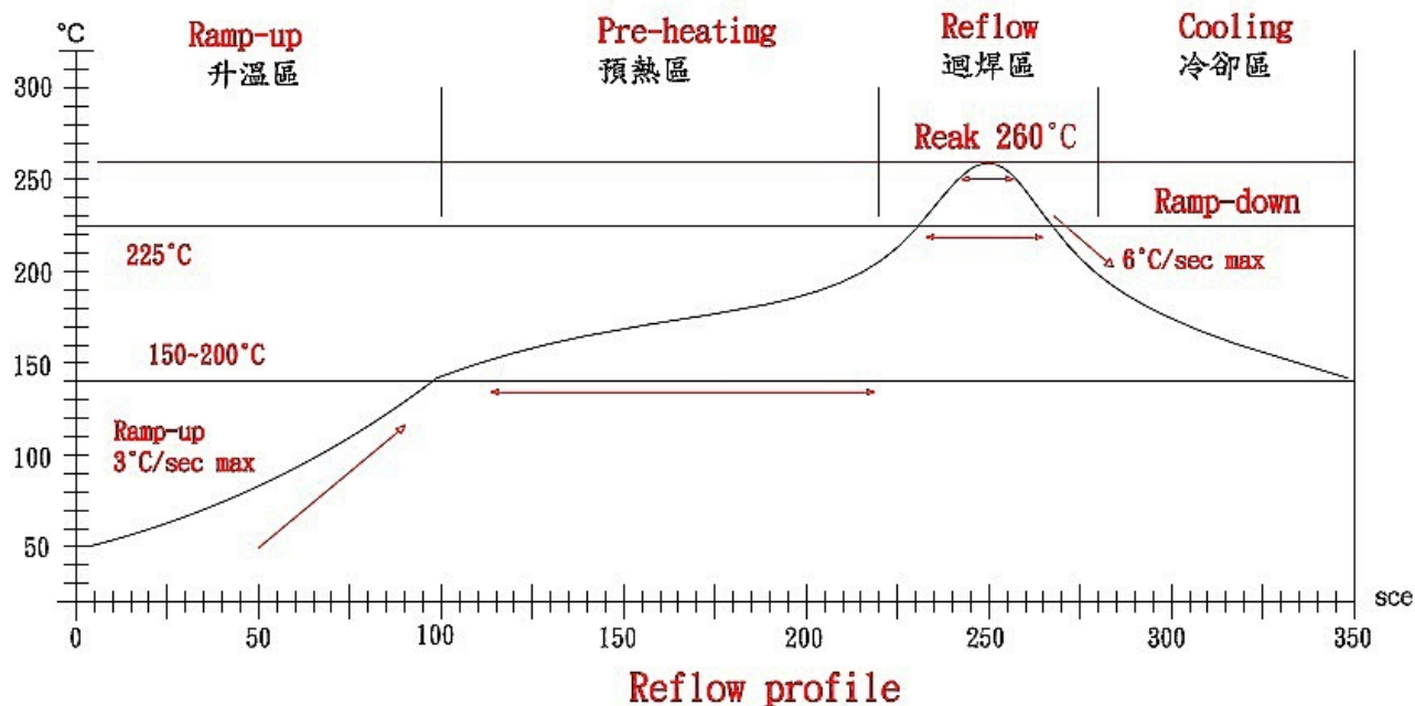
Lead-Free(LF)標準溫度分析範圍
