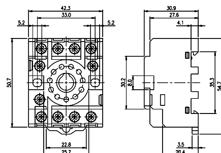
CS113AN
