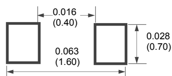
0402 Size
