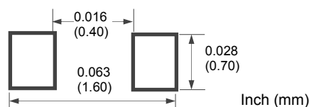
0402 Size
