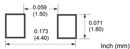
1206 Size
