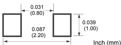
0603 Size
