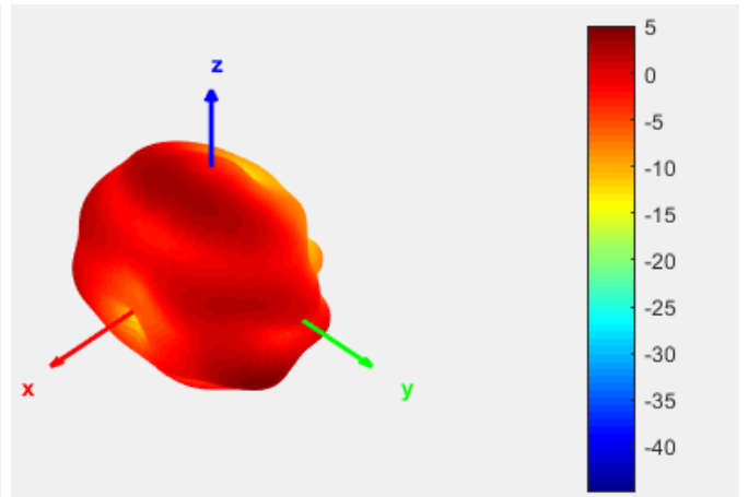
8GHz
