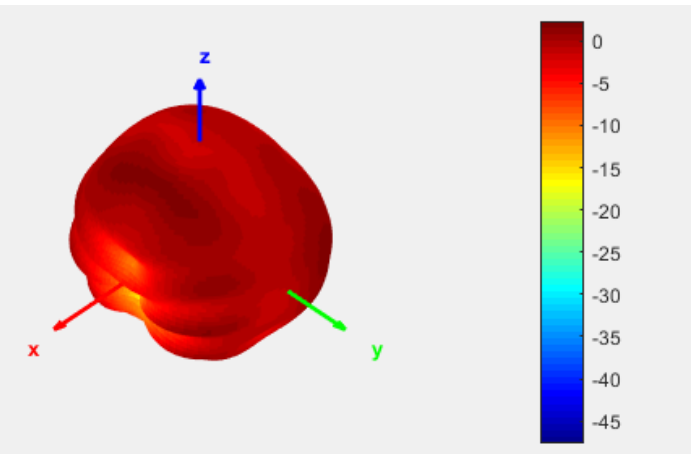
8GHz
