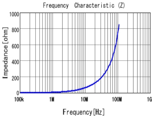
■ LQH2HPZ1R0MDR |Z|
