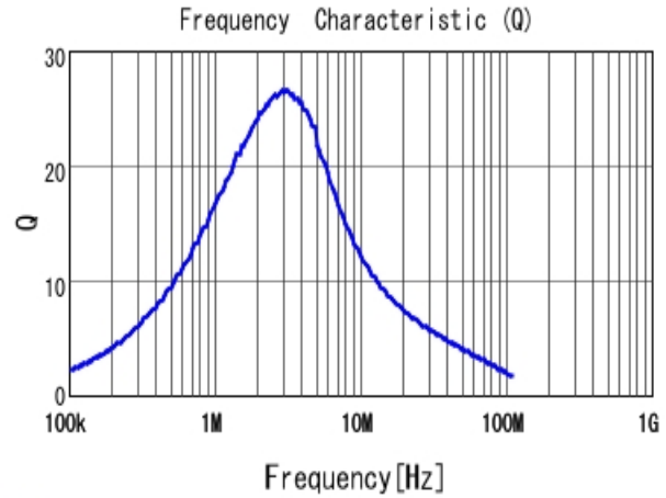
■ LQH2HPZ1R0MDR Q
