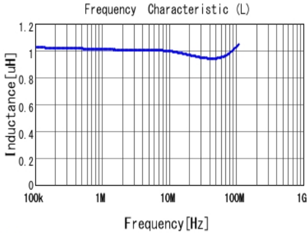
■ LQH2HPZ1R0MDR L
