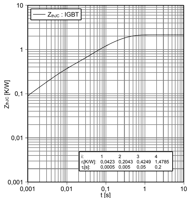
瞬态热阻抗 IGBT, 三电平 transient thermal impedance IGBT,3-Level
