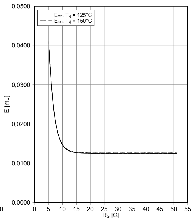
Schaltverluste Diode, Hochsetzsteller (typisch) switching losses Diode, Boost (typical) E_{rec} = f(R_G) I_F = 30 A , V_{CE} = 400 V
