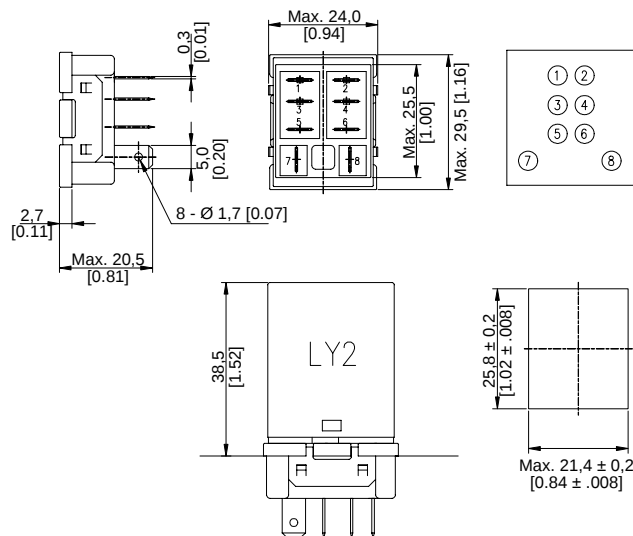
FIGURE 10. SZX-SLB-08
