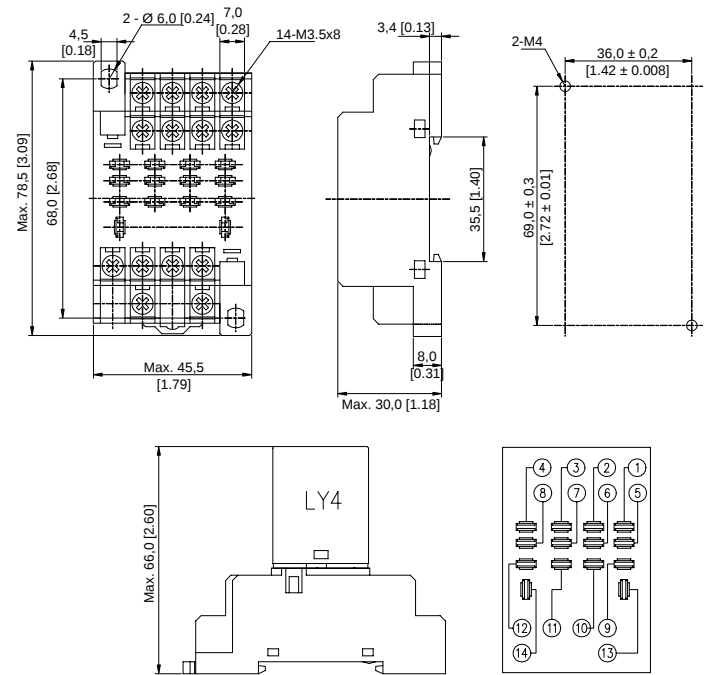
FIGURE 11. SZX-SLB-14
