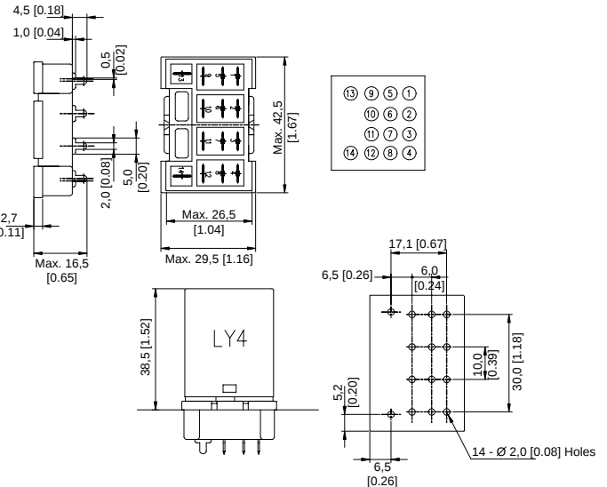
FIGURE 13. SZX-SLB-14P
