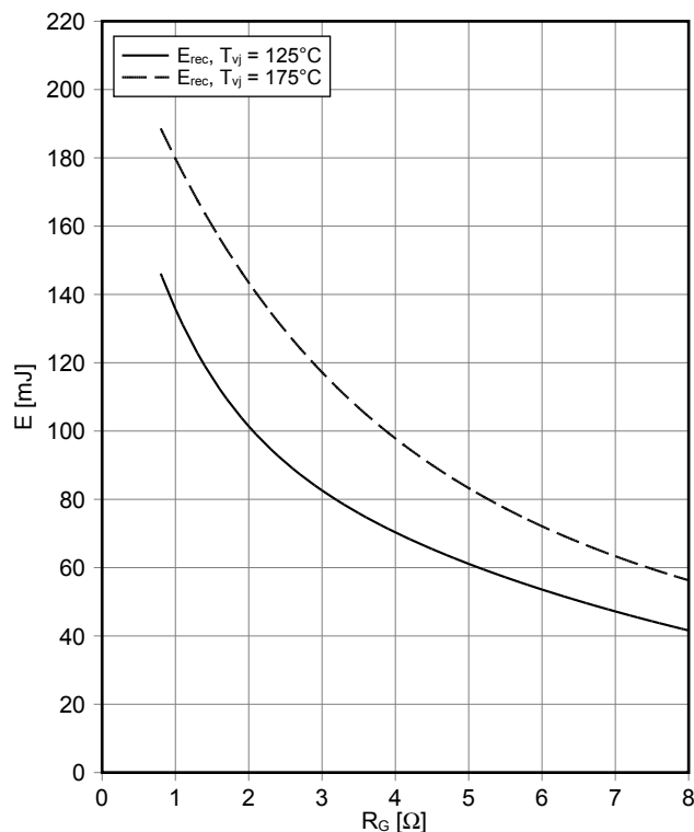
スイッチング損失 Diode、インバータ (Typical) switching losses Diode, Inverter (typical) E_{rec} = f(R_G) I_F = 1800 \text{ A} , V_{CE} = 600 \text{ V}
