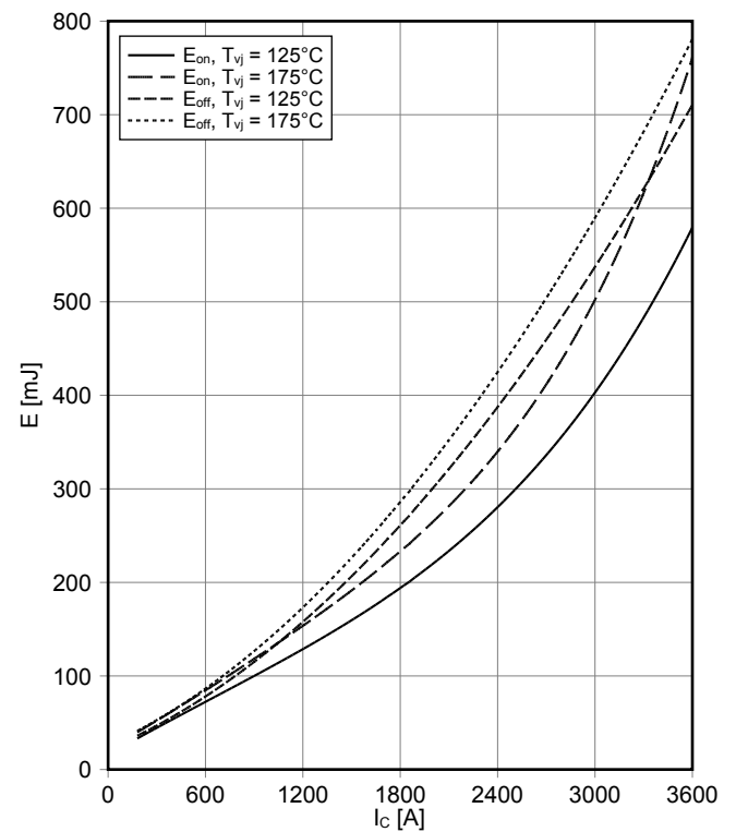
スイッチング損失 IGBT- インバータ (Typical) switching losses IGBT, Inverter (typical) E_{on} = f(I_C) , E_{off} = f(I_C) V_{GE} = \pm 15\text{ V} , R_{Gon} = 0.82\ \Omega , R_{Goff} = 0.82\ \Omega , V_{CE} = 600\text{ V}
