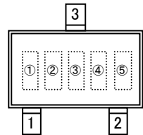
SOT-323-3A
