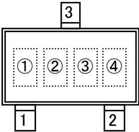
SOT-523
