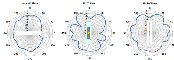
5500 MHz
