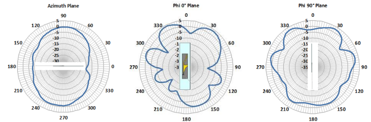
5150 MHz
