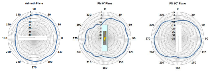
2300 MHz
