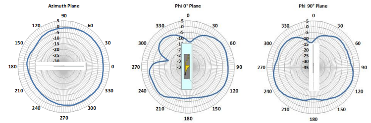
2595 MHz
