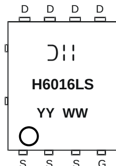
PowerDI5060-8
