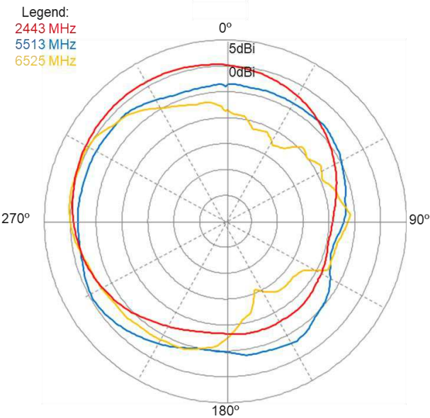
Elevation 2
