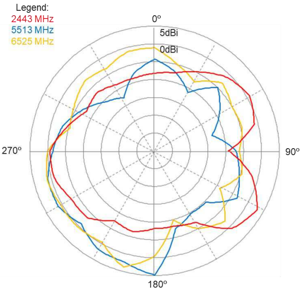
Elevation 2
