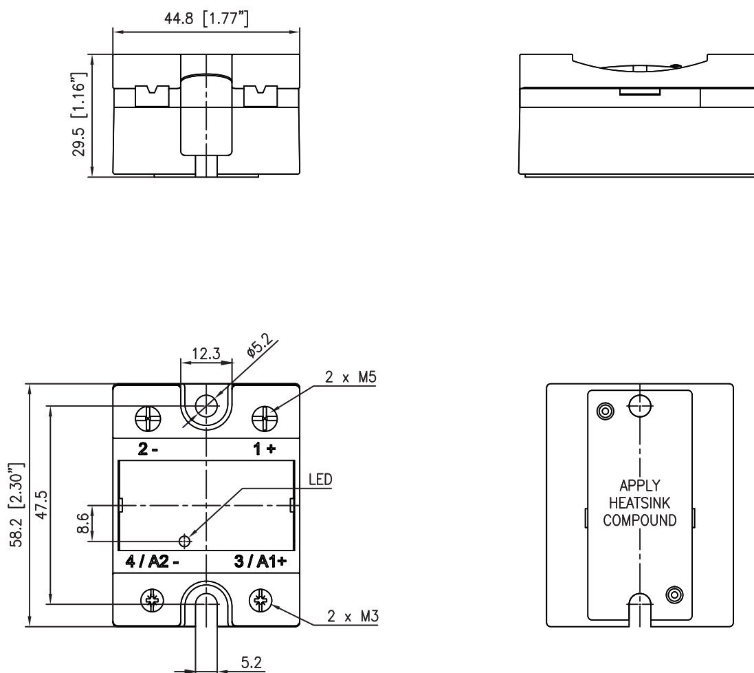
Fig. 1 RM1D dimensions
