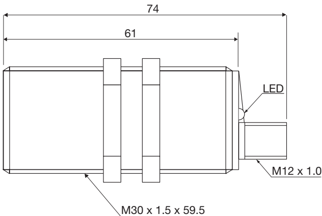
Fig. 8 Plug CA30CAF...M1IO
