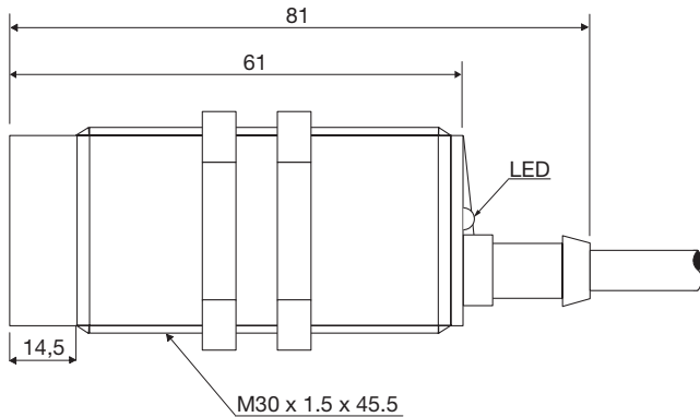
Fig. 7 Cable CA30CAN...A2IO
