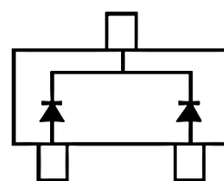
BAT54C
