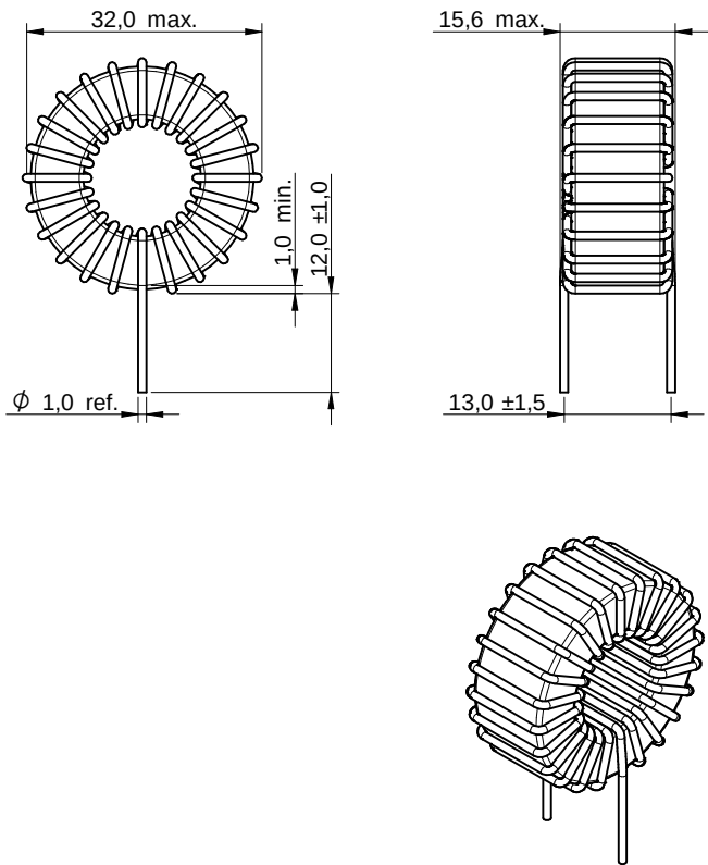
Scale - 1:1
