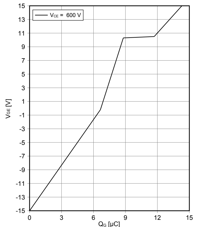
Gateladungs Charakteristik IGBT, Wechselrichter (typisch) gate charge characteristic IGBT, Inverter (typical)
