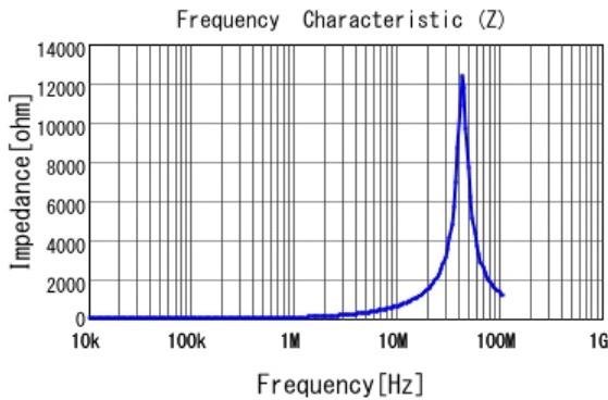
■ LQH2HPZ100MJR |Z|
