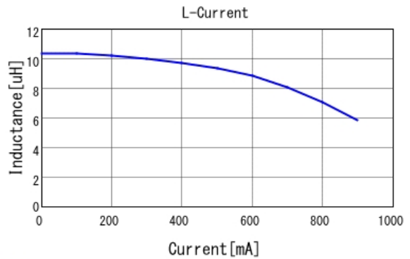
■ LQH2HPZ100MJR L-Current 20degC
