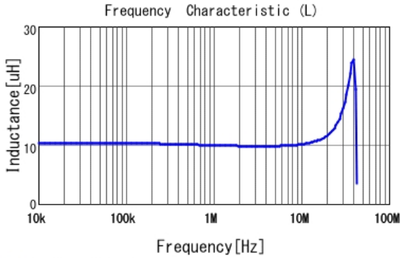
■ LQH2HPZ100MJR L
