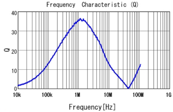
■ LQH2HPZ100MJR Q
