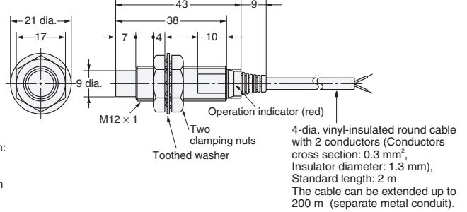
Fig. 12: E2E-X5MY□
