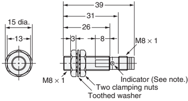
Fig. 28: E2E-X2D□-M3G/E2E-X1R5E□-M3/F□-M3
