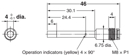
E2E-S05N03-MC-□□
