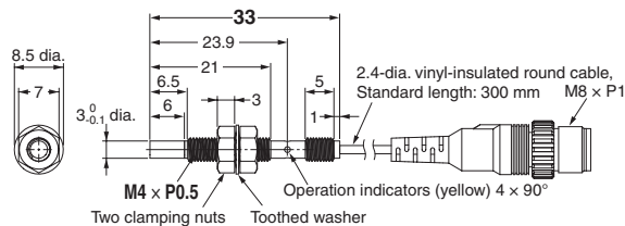
E2E-S04N02-CJ-□□
