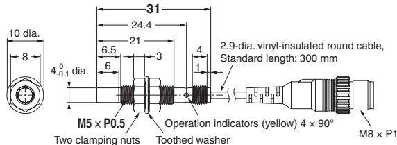
E2E-S05N03-CJ-□□
