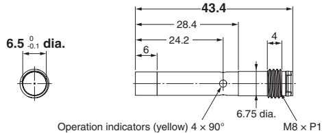
E2E-C06N04-MC-□□
