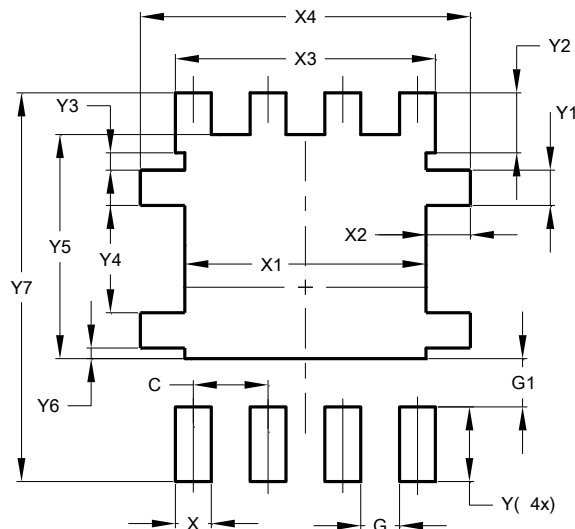
PowerDI5060-8
