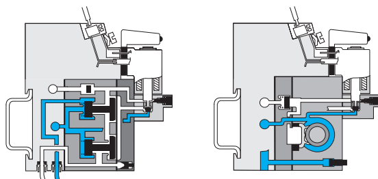
4/2 monostable module
