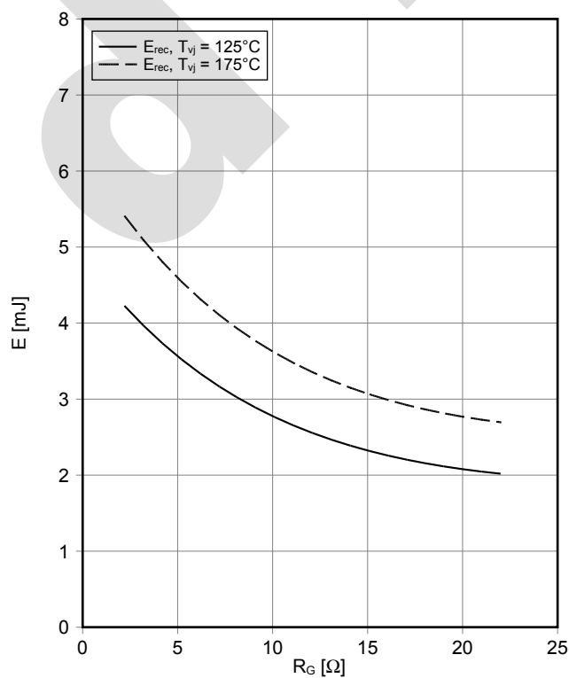
Schaltverluste Diode, Wechselrichter (typisch) switching losses Diode, Inverter (typical) E_{rec} = f(R_G) I_F = 75 \text{ A} , V_{CE} = 600 \text{ V}
