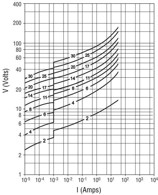
Model Size 0603 - (ZV 2 M 0603 300 ~ ZV 30 K 0603 300)
