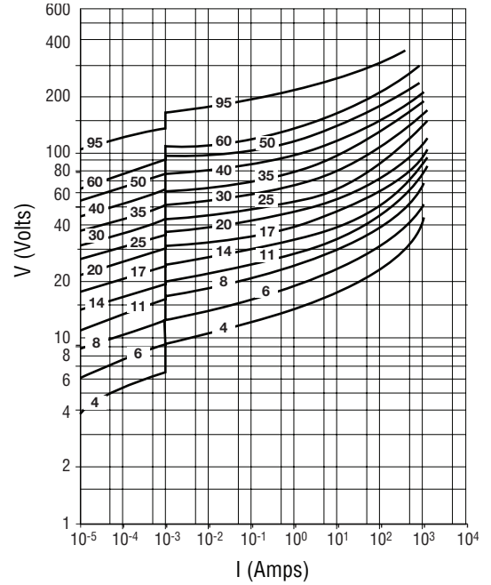
Model Size 2220 - (ZV 4 M 2220 xxx ~ ZV 95 K 1210 xxx)
