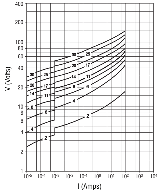
Model Size 0805 - (ZV 2 M 0805 xxx HT ~ ZV 30 K 0805 xxx HT)
