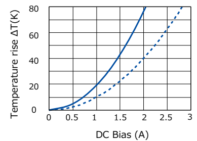
[ ETQP5M101YGM ]
