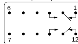
219BXP (DPDT)
