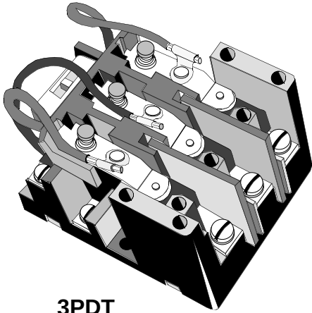
3PDT
