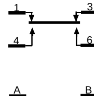
SPDT-NC-NO- (DB-DM)
