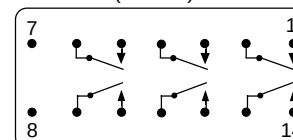
219FXXP (6P-NO)
