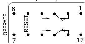
B255XBXP (DPDT)
