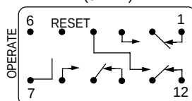
B255XCXP (3 PDT)
