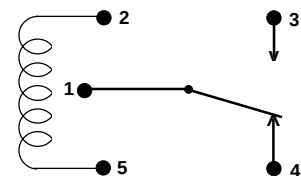
SPDT
