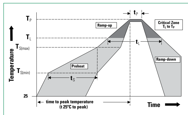
Soldering Parameters
