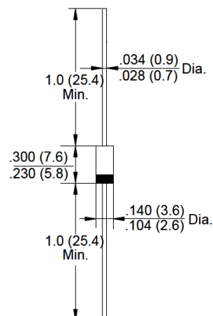
DO-204-AC (DO-15)
