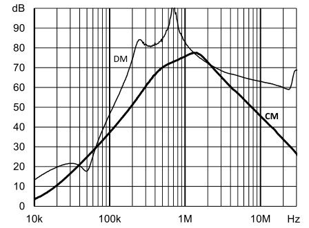
FN 3288-50-53-C21-R65
