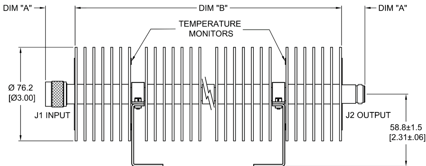
Attenuator Dimensions
