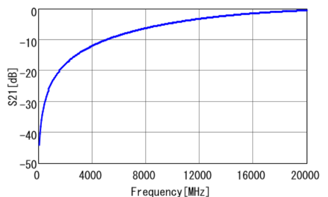
S Parameter S21
