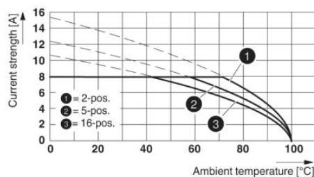
Type: MCV 1,5/...-ST-3,5 AU with MCV 1,5/...-G-3,5 AU
