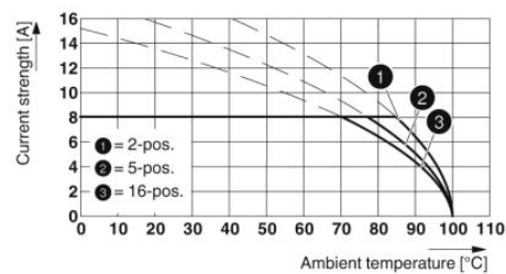
Type: MC 1,5/...-ST(F)-3,5 AU with MCV 1,5/...-G(F)-3,5 AU
