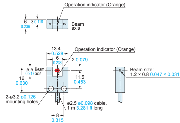
PM-U25
