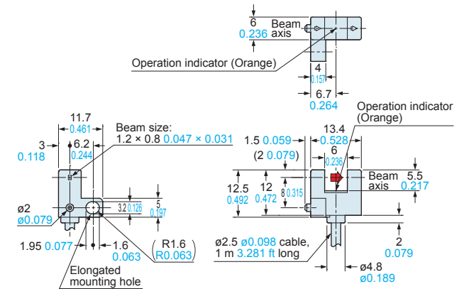
PM-F25
