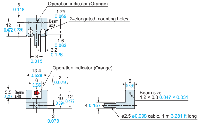
PM-L25
