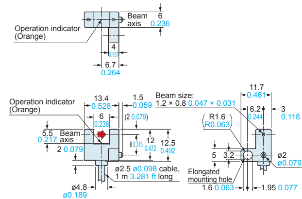
PM-R25
