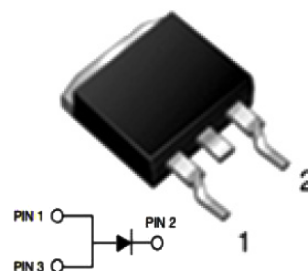
TO-263AB
